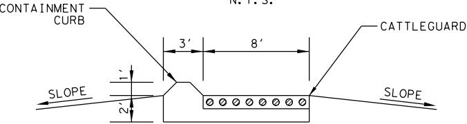
PERIMETER CONTAINMENT BERM N. T. S.
