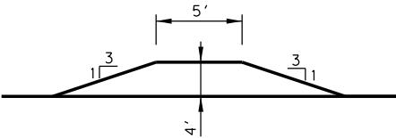
PERIMETER CONTAINMENT BERM N. T. S.
